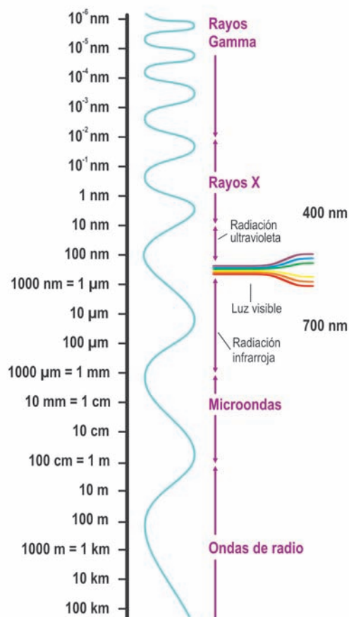
Figura 6. Espectro electromagnético.
