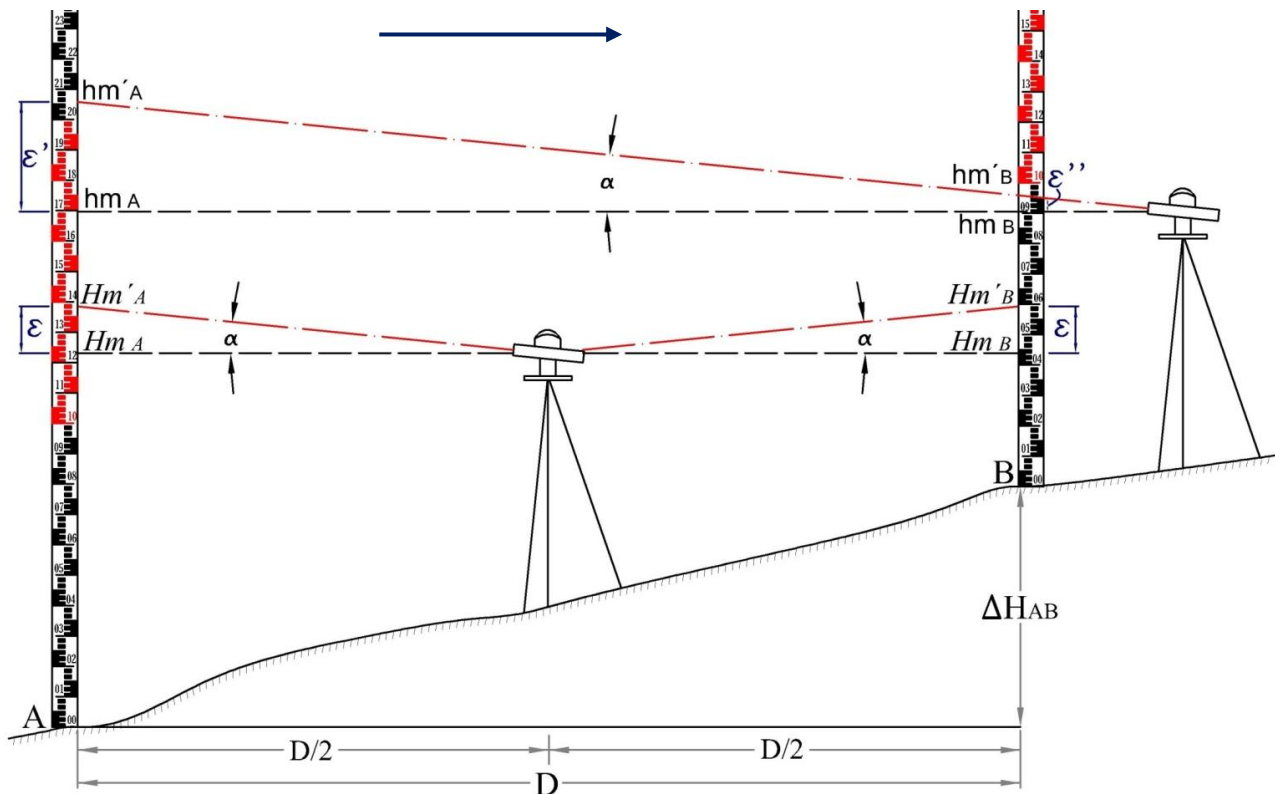
Figura 10-a: Detección del error de colimación en un nivel de anteojo (Procedimiento valido tanto para aparatos Automáticos y como de Línea).
