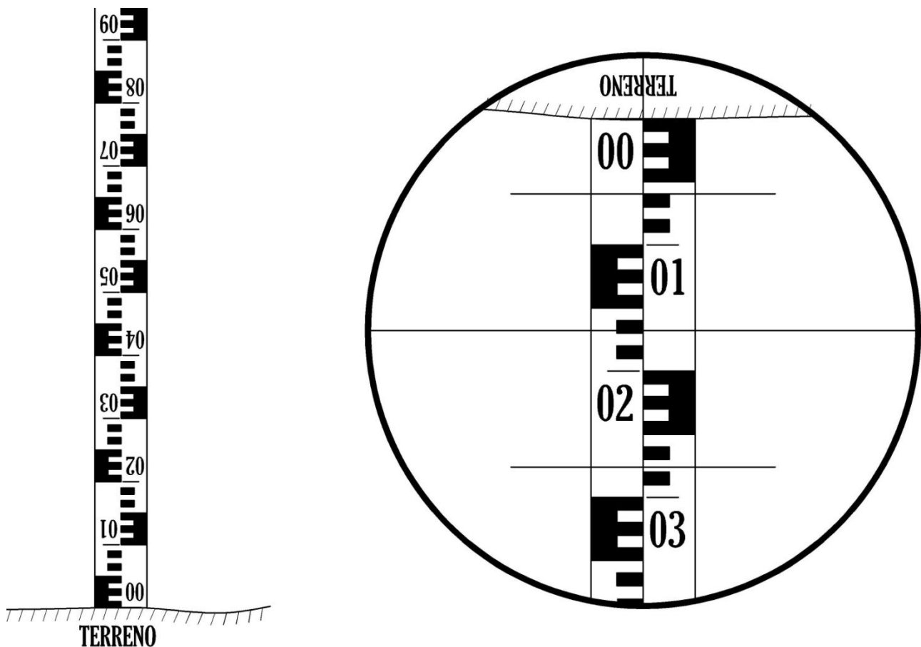
Figura 6-c: Izquierda: Mira con graduaciones invertidas. Derecha: colimación a mira de graduaciones invertidas con un nivel de línea. Lectura de hilo medio (Hilo Horizontal principal) 0,168. Los décimetros (01) se leen directamente, los centímetros (6) se cuentan tomando como referencia la graduación tipo “E”, y los milímetros (8) se estiman. Las lecturas de hilo superior e inferior respectivamente son 0,060 y 0,276. Nótese que para este tipo de lectura, el hilo superior es menor que el hilo inferior ya que la imagen está invertida.
