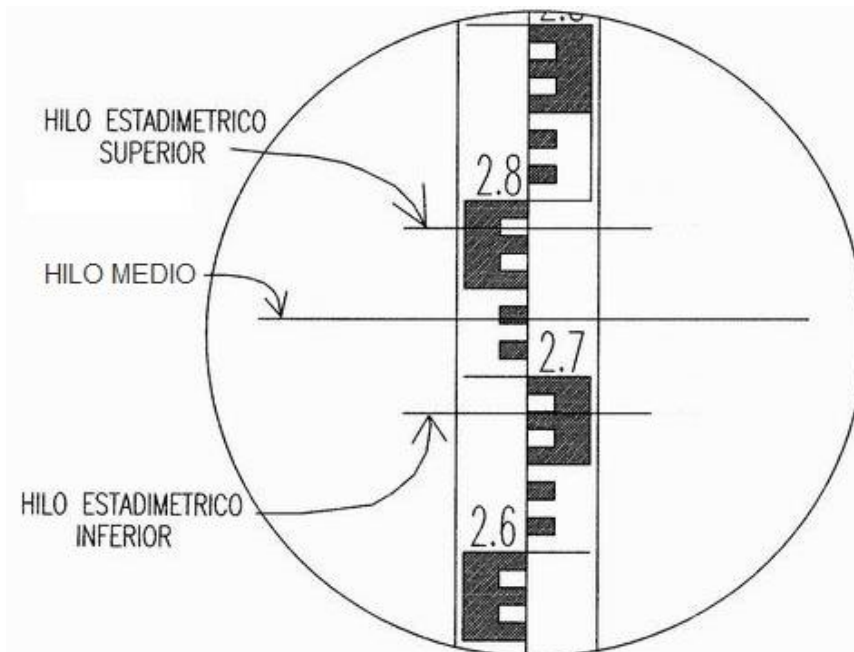
Figura 13: Hilo superior= 2,785 Hilo medio= 2,732 Hilo inferior= 2,679
