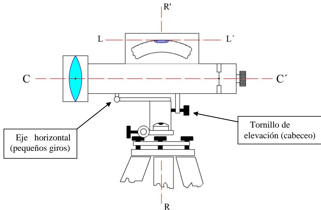
Figura 4: Esquema de nivel de línea. LL' debe ser paralelo a CC' , de ese modo cuando LL' es horizontal (burbuja centrada) CC' también lo es.
