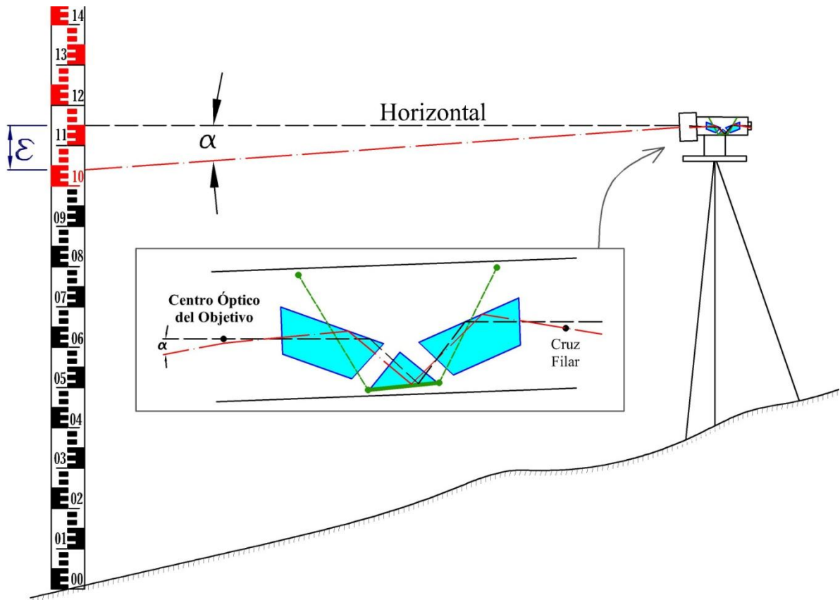
Figura 9: Error de colimación en un nivel Automático. La posición del retículo no es la correcta, por lo tanto la lectura de hilo medio no se corresponde con una visual horizontal.
