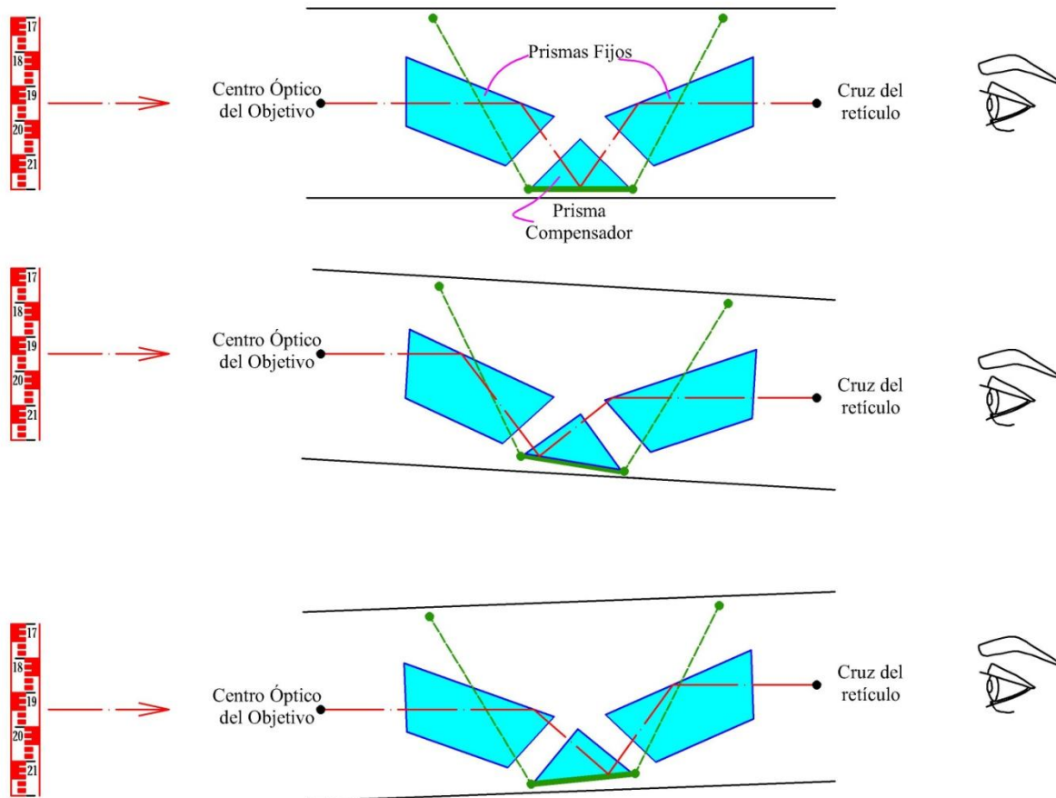
Figura 5b: Esquema del sistema compensador de un nivel Automático en tres posiciones diferentes. Calado el nivel esférico, el sistema compensador estará dentro de su rango de trabajo. Entonces, la visual horizontal que pasa por el centro óptico del objetivo, por acción del compensador, atravesará siempre la cruz filar del retículo. Imagen: Wolf y Ghilani – Topografía – 11 edición, 2008 - página 90.
