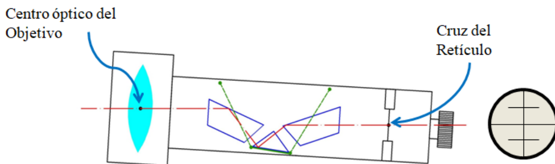
Figura 5-a: Esquema de un nivel Automático. Estando calado el nivel esférico, el anteojo no está perfectamente horizontalizado. El compensador automático provoca que la visual que atraviesa la cruz del retículo sea horizontal.
