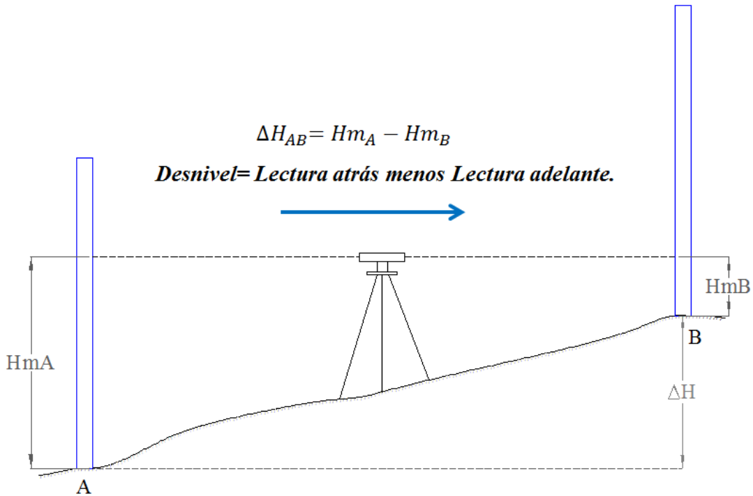
Figura 7: Medición geométrica del desnivel entre dos puntos A y B. Miras verticalizadas sobre los puntos A y B, y visual horizontal dada por el nivel de anteojo.
